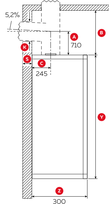
vista lateral
